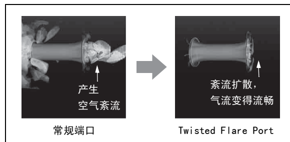
两端口的空气紊流产生噪音
